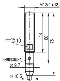
Габаритный чертёж
